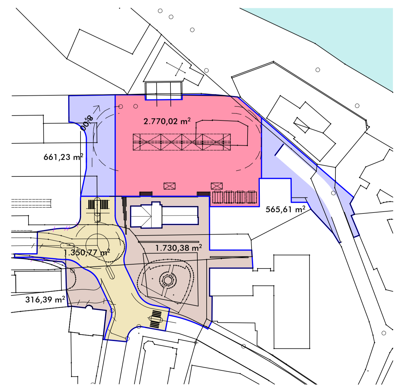
Übersicht Bauabschnitte (M 1/1000) Ausbau Münchner Straße - Im Hag (St 2359) / Kreisverkehr Neubau eines Busbahnhofes am Altstadtbahnhof Neugestaltung Bahnhofplatz
